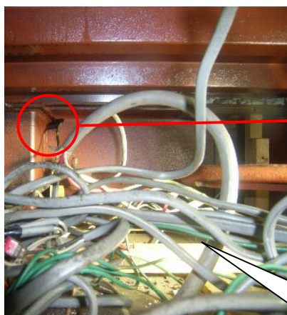
壁内部の電気配線の状況
