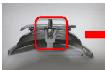
ボンベ上部切断写真
