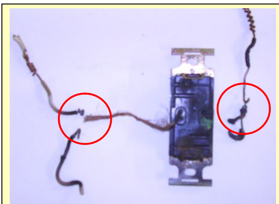
不適切な接続部分
